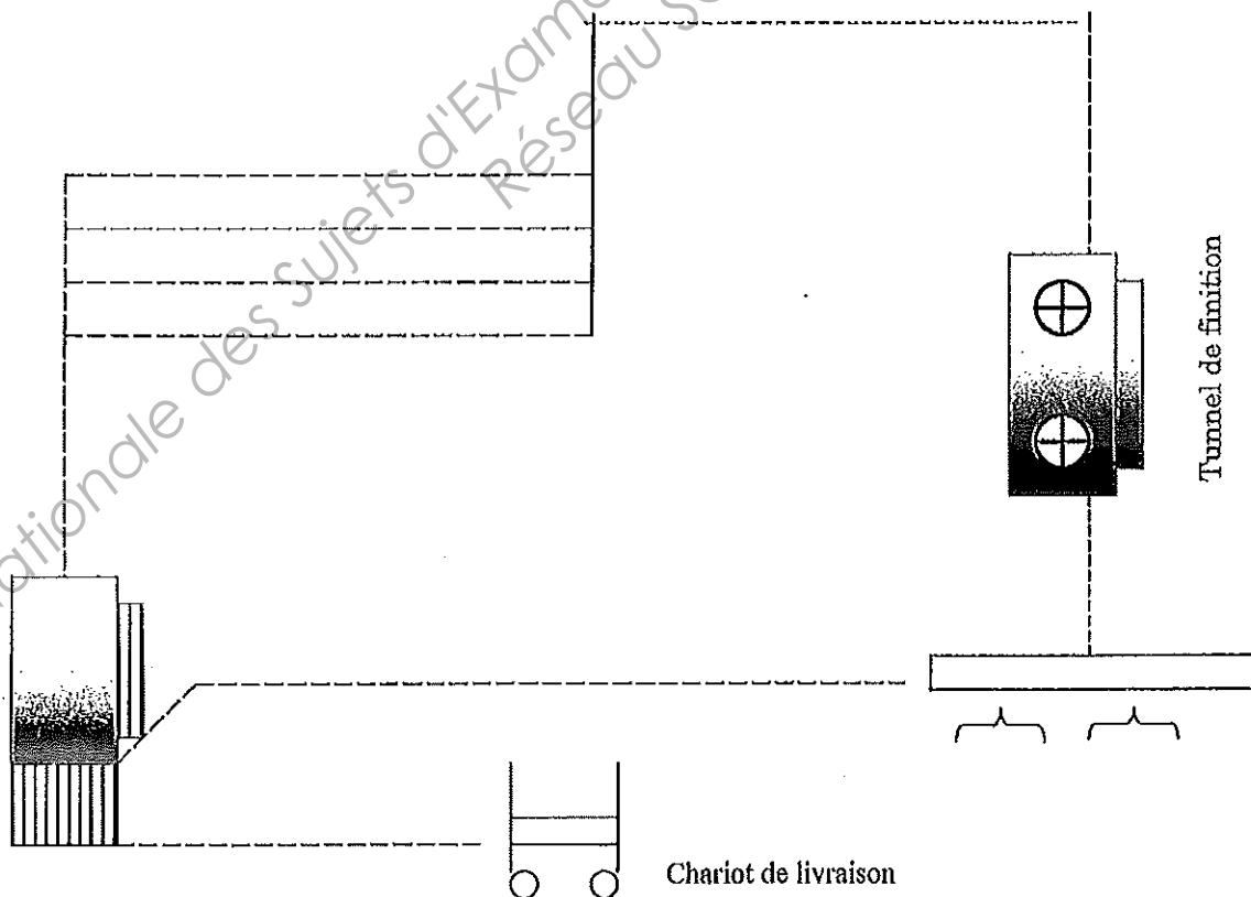
Schéma d'implantation
